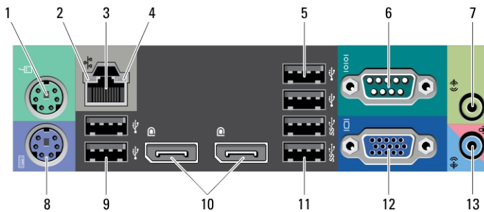
Αριθμός 2. Όψη πίσω πλευράς
